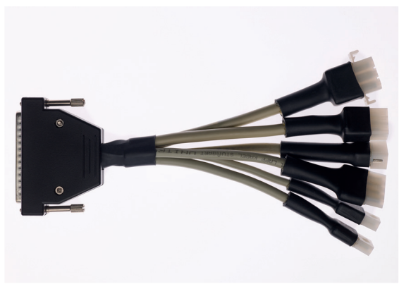
Sechs Kabel – eine Seite mit Steckern versehen, Flachkabel mit Crimpverbindern. Die andere Seite zu einem einzigen D-Sub-Stecker zusammengefasst.
