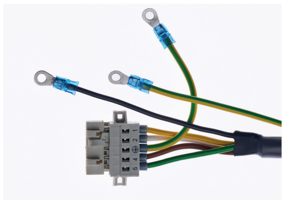
Multicore-Kabel – auf die Adern gecrimpte Aderendhülsen, montierter Stecker und zusätzliche Adern mit gecrimpten Kabelschuhen.
