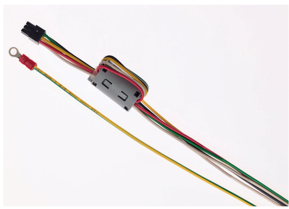
Kabel mit Stecker, Kabelschuh und Ferritkern.
